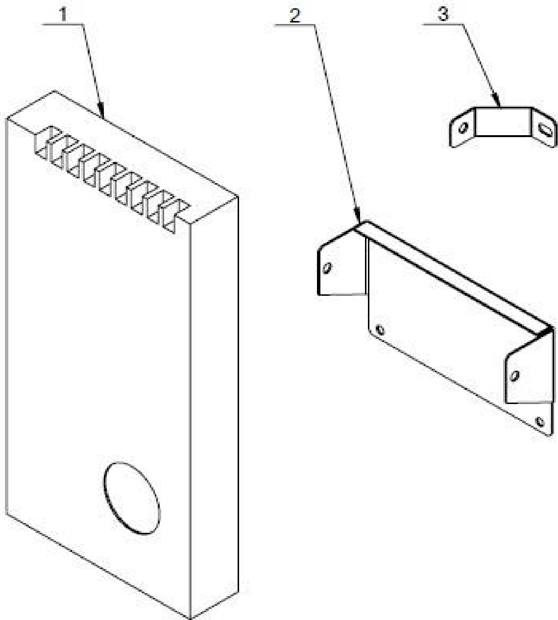
b - Блок живлення 24 В в зборі
