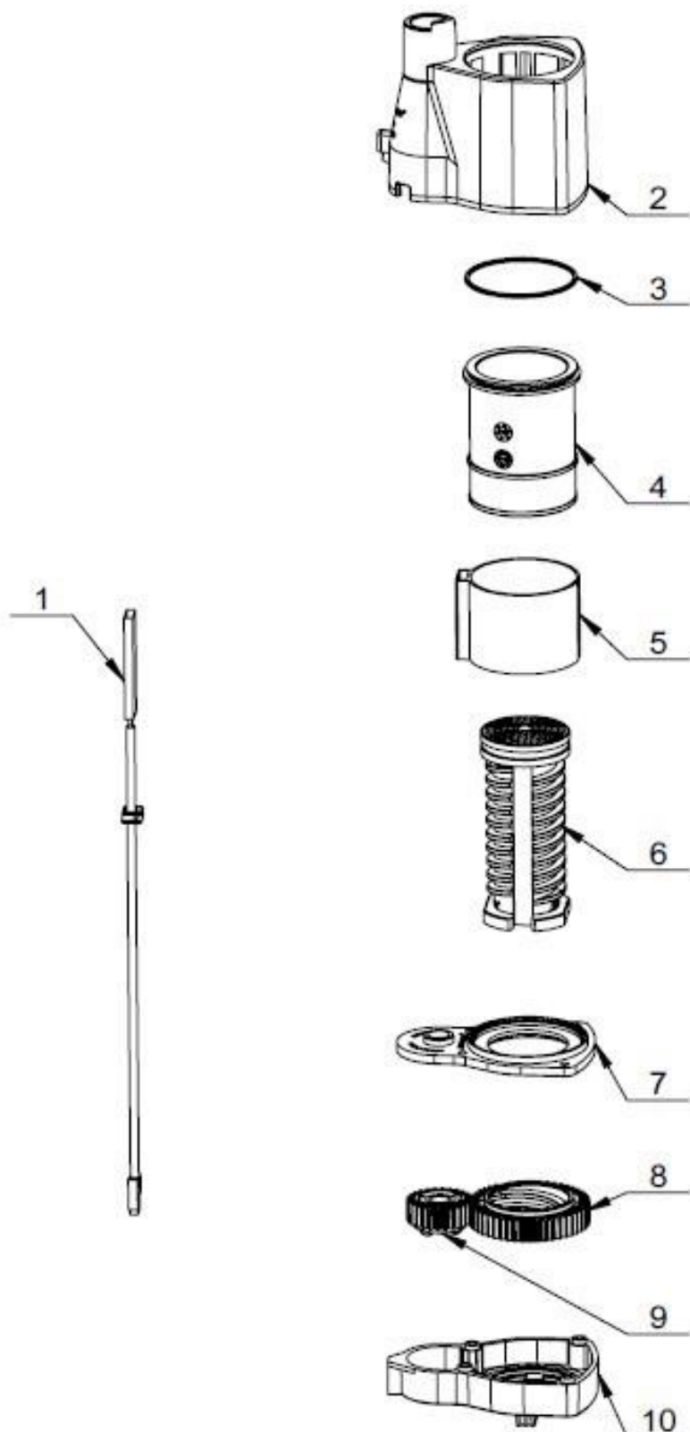
3111055500 Заварювальня камера 14 г в зборі
